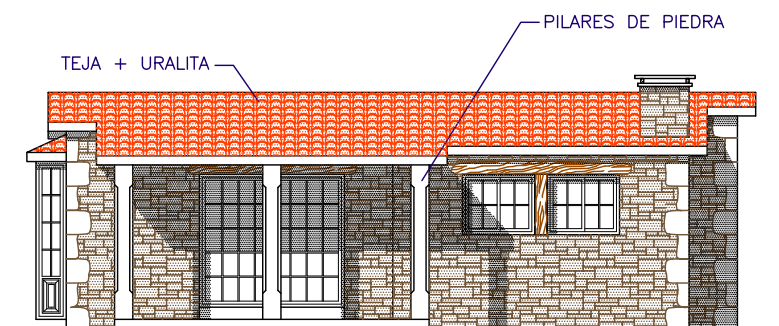
ALZADO SUR
